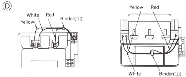
H300C, H400
